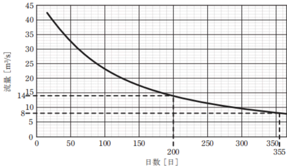
図 流況曲線
